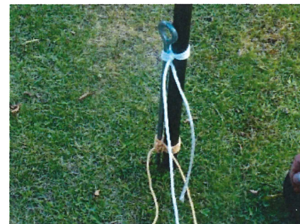
支柱の固定方法
